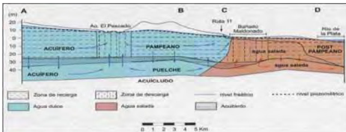
Figura 11: Acuíferos subterráneos presentes en la región 19
