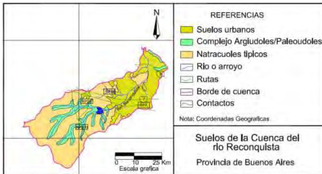
Figura 12: Suelos Cuenca Reconquista
