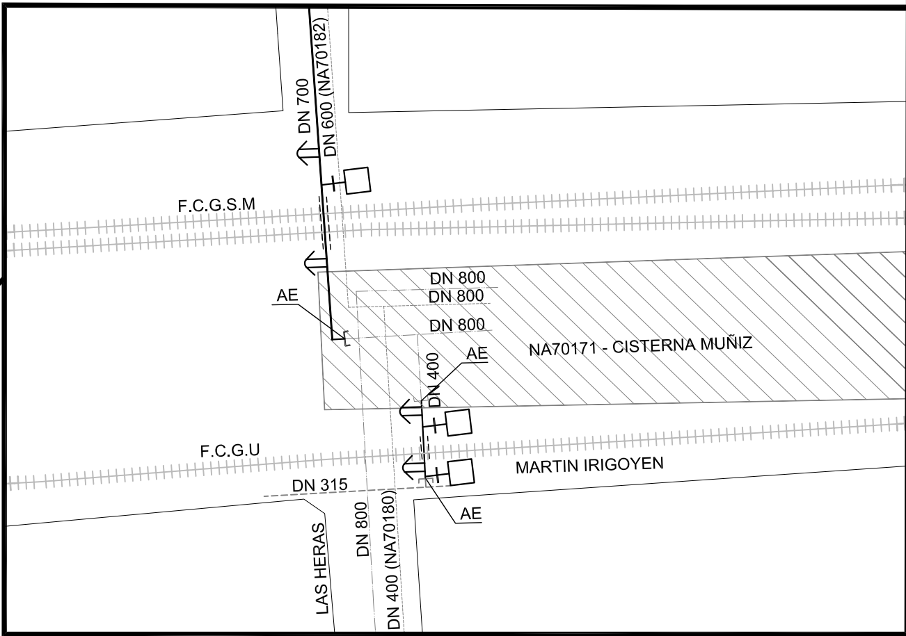
DETALLE EMPALME CISTERNA MUÑIZ (Esc. 1:1000)
