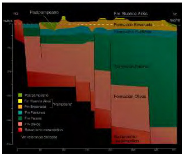
Figura 5: Esquema de corte estratigráfico suelo – subsuelo
